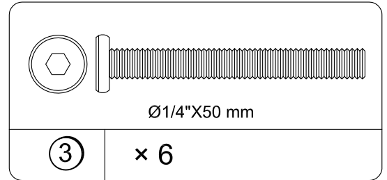
Bolt TKX1102
